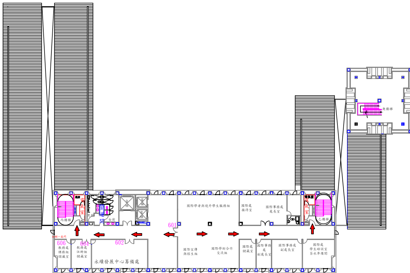
行政大樓6樓緊急逃生避難平面圖
