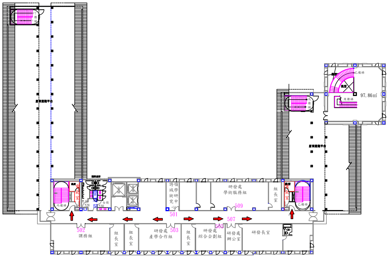
行政大樓5樓緊急逃生避難平面圖
