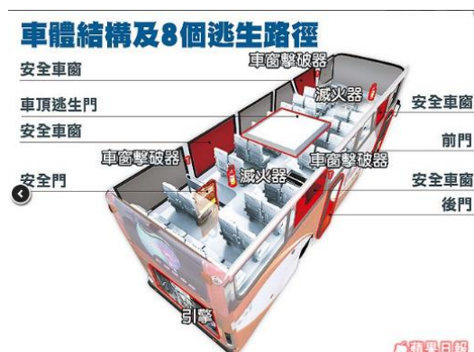
< 圖二十二：車體結構及逃生路徑 >
