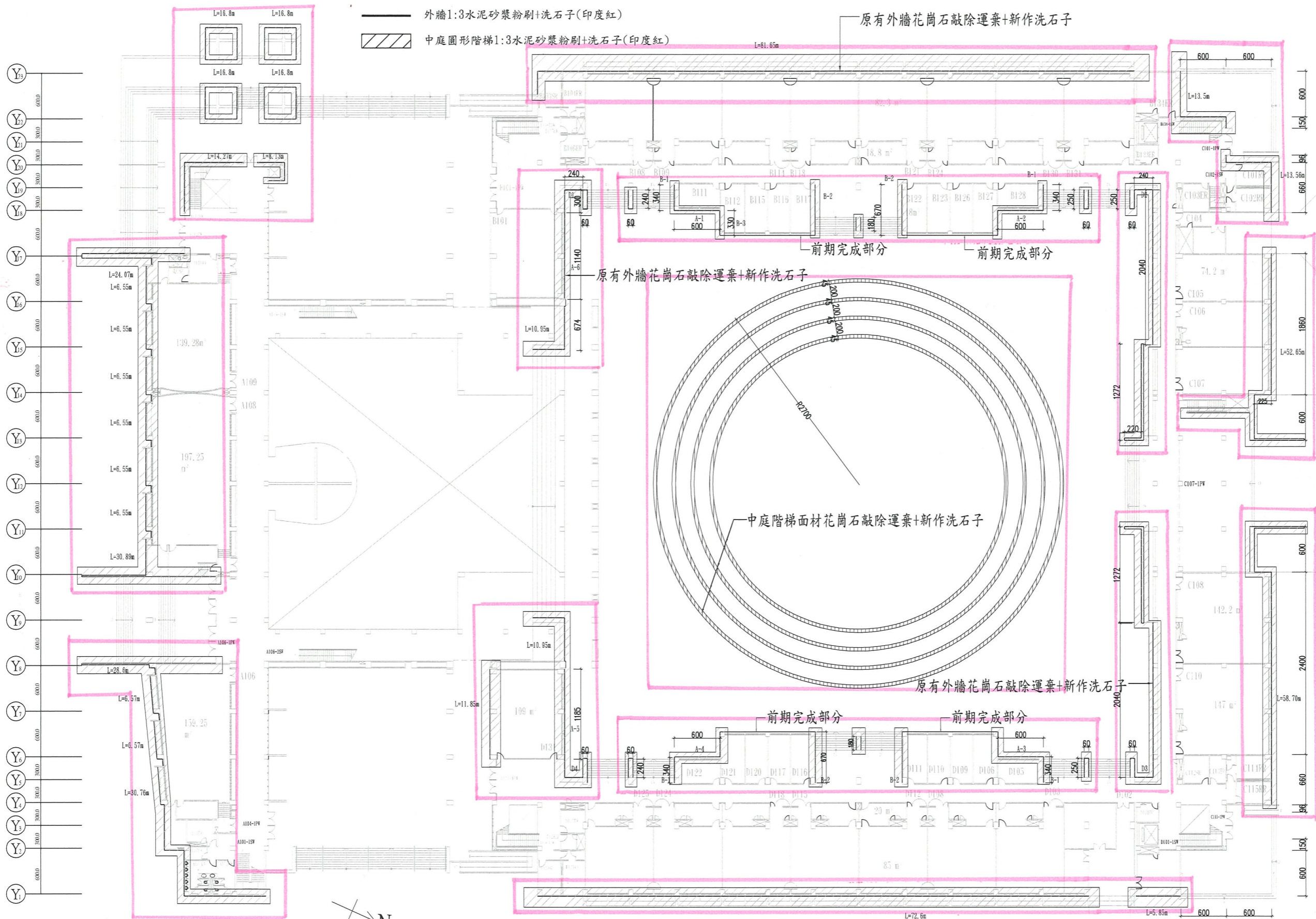
理工一館一層改善平面圖 S=1/1000
