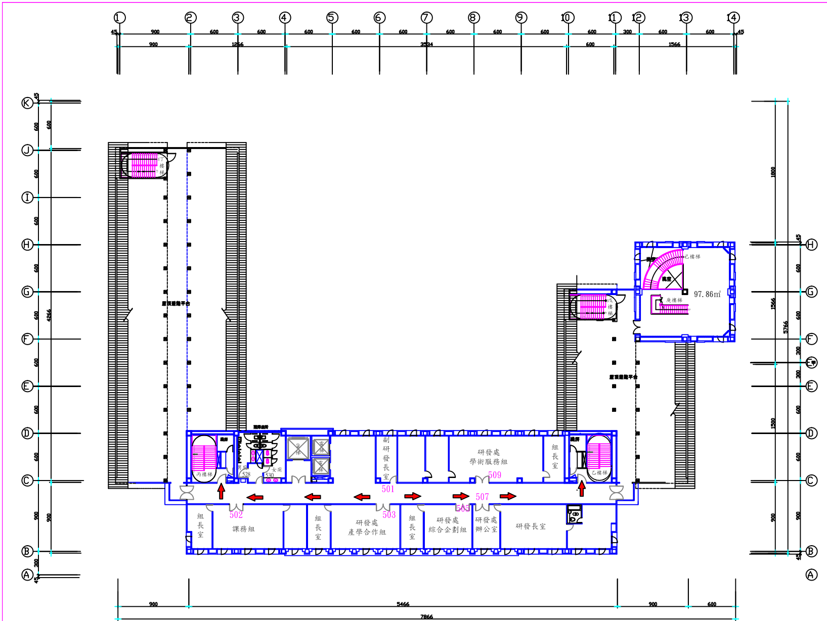
行政大樓5樓平面圖暨避難逃生路線圖
