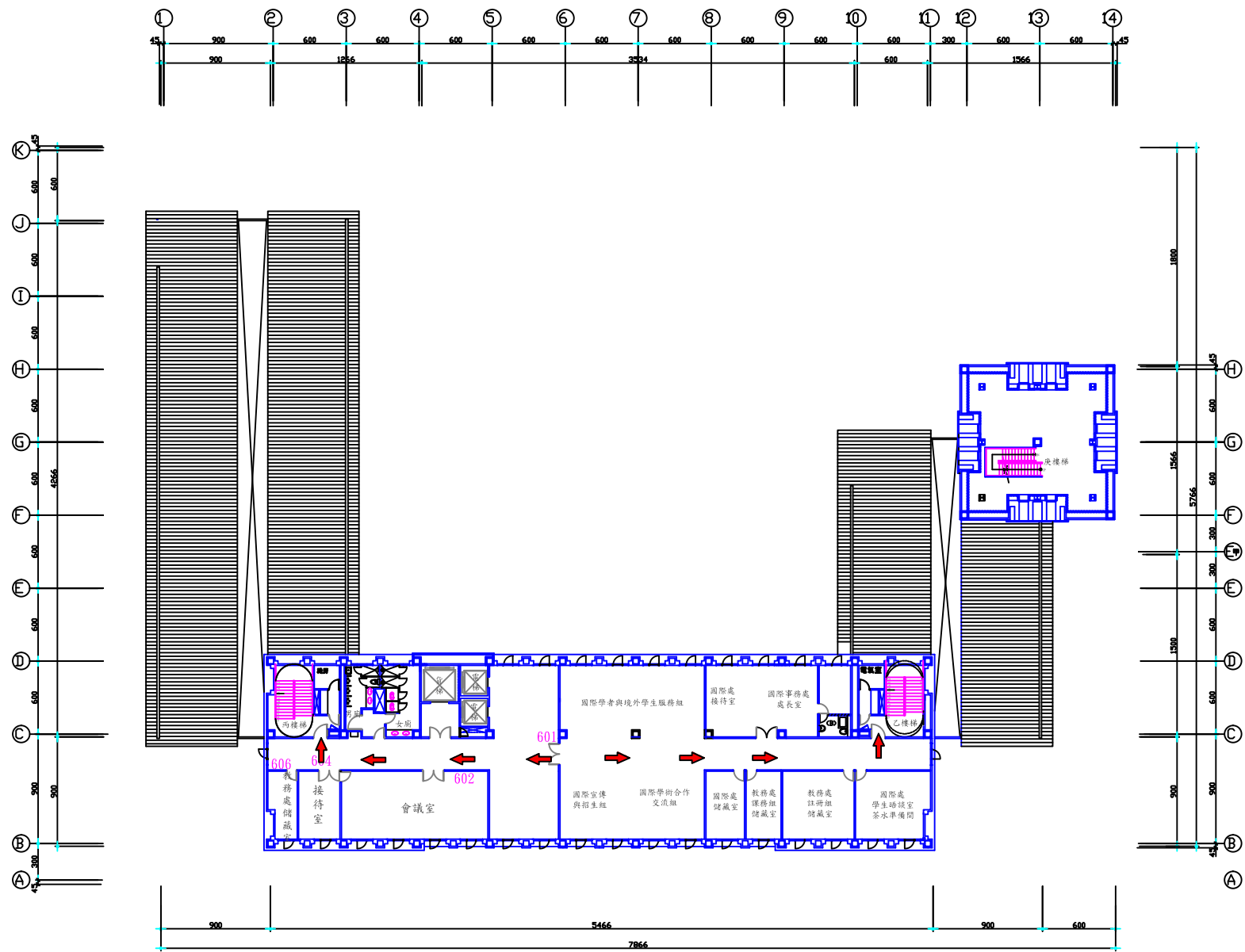
行政大樓6樓平面圖暨避難逃生路線圖
