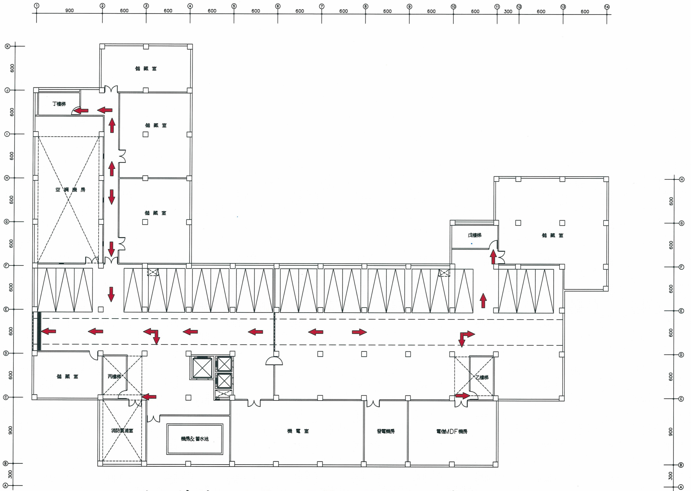
行政大樓地下室平面圖暨避難逃生路線圖
