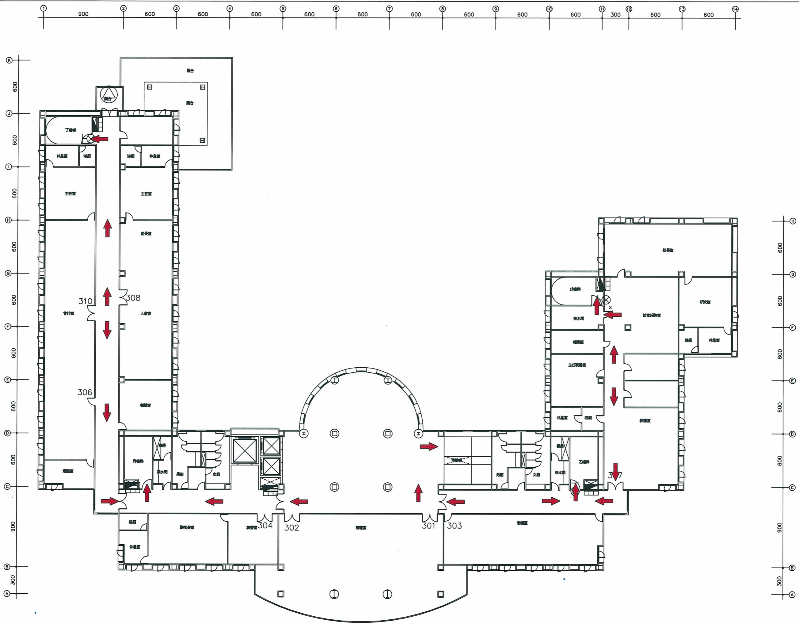
行政大樓3樓平面圖暨避難逃生路線圖
