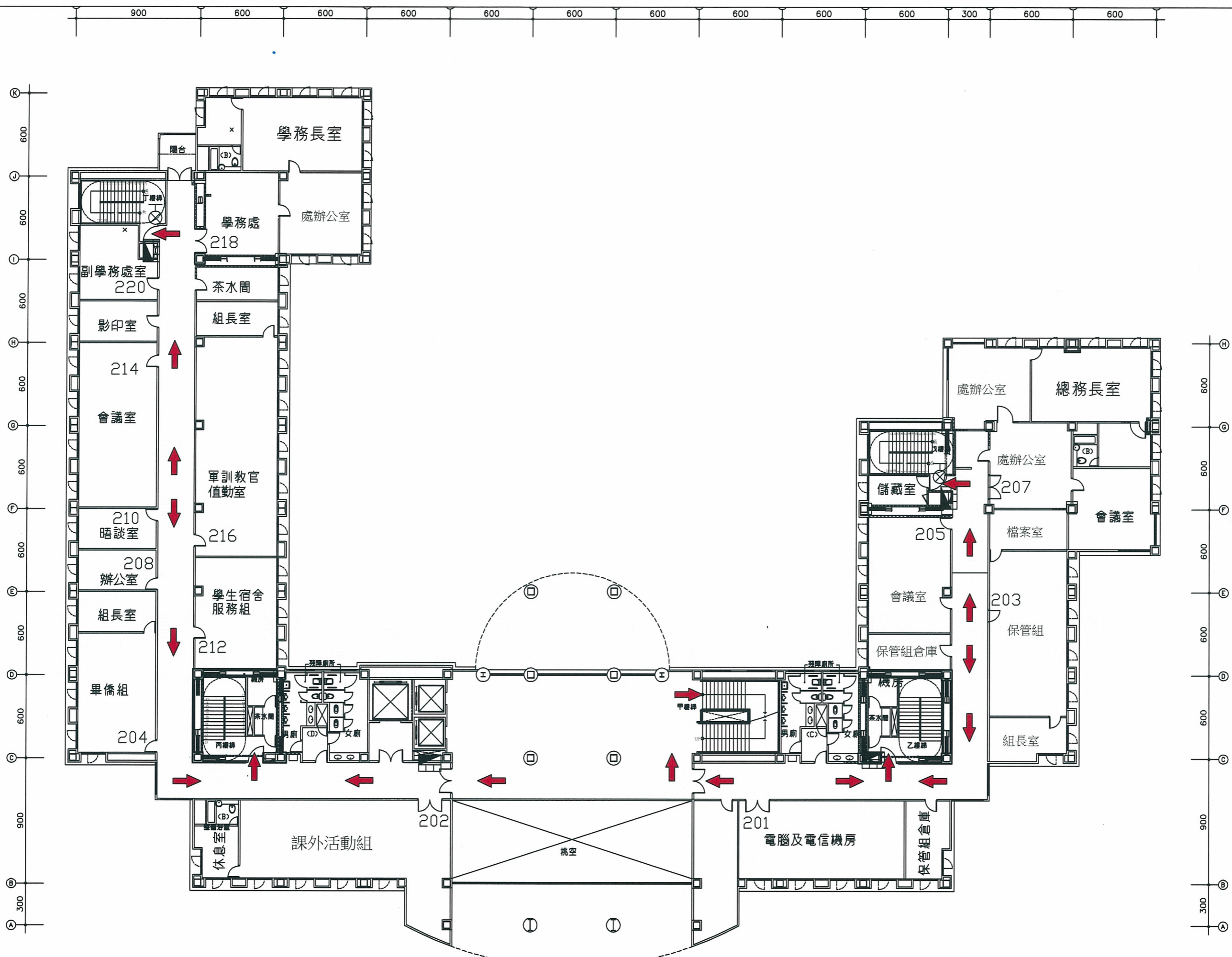
行政大樓2樓平面圖暨避難逃生路線圖
