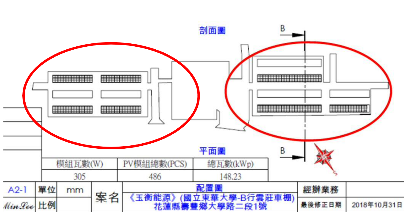
附圖四 行雲莊機踏車車棚吊掛位置示意圖
