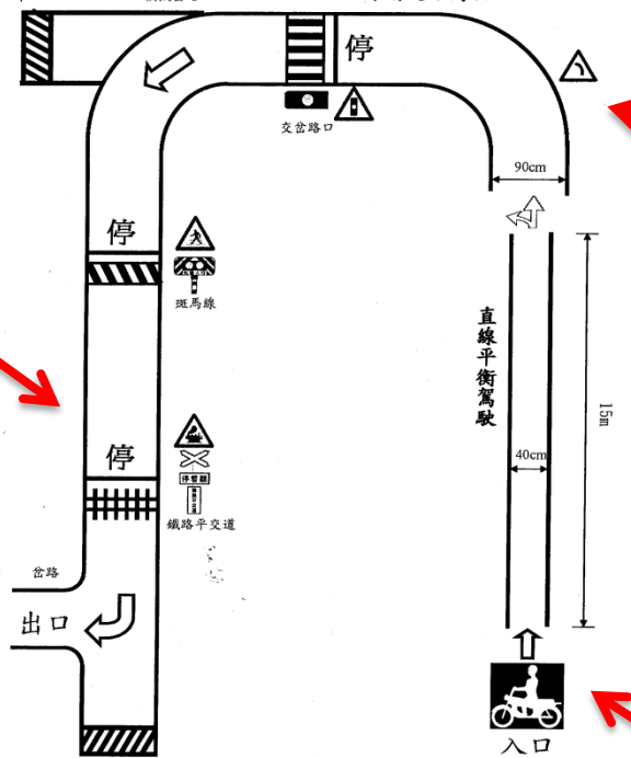
(六)普通重型機車考驗場配置參考圖 普通重型機車考驗場配置參考圖
